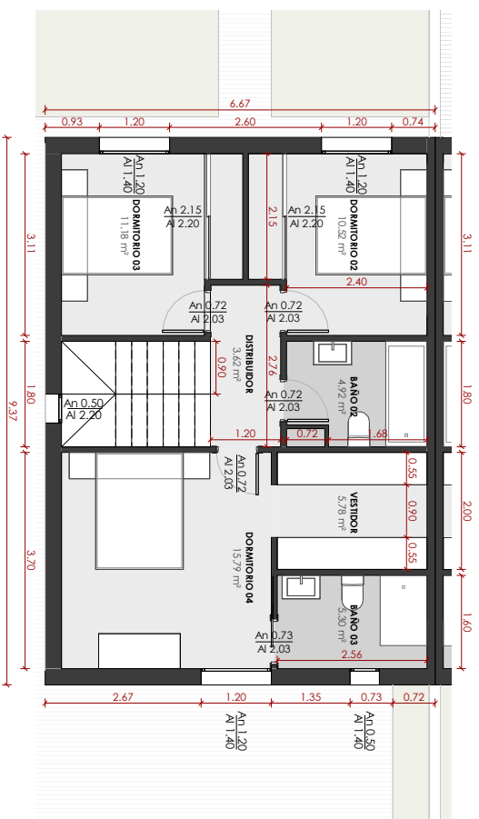
PLANTA PRIMERA E-1175
