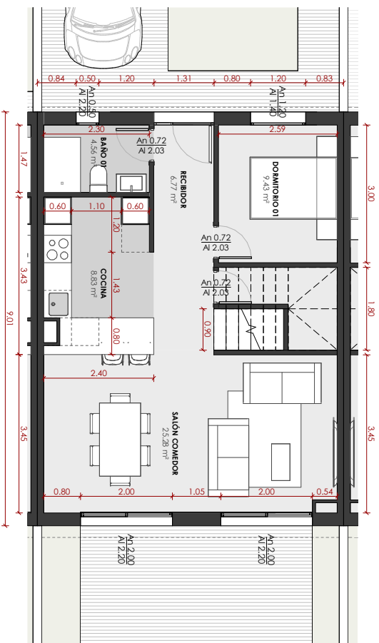
PLANTA BAJA E-1175
