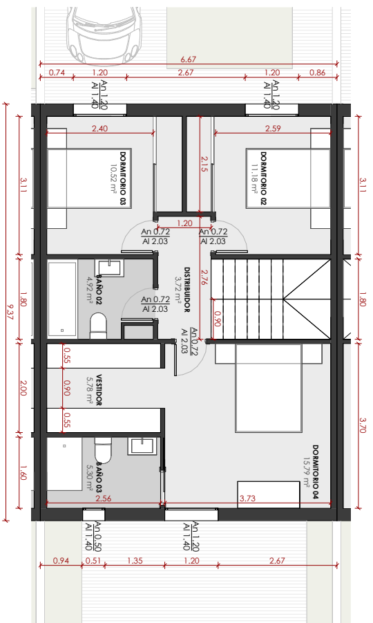
PLANTA PRIMERA E-1175
