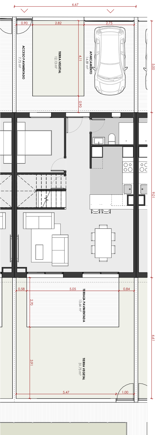
PLANTA BAJA - E - 1/75
