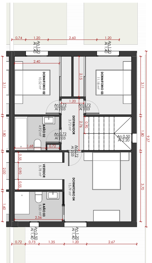
PLANTA PRIMERA E-1175
