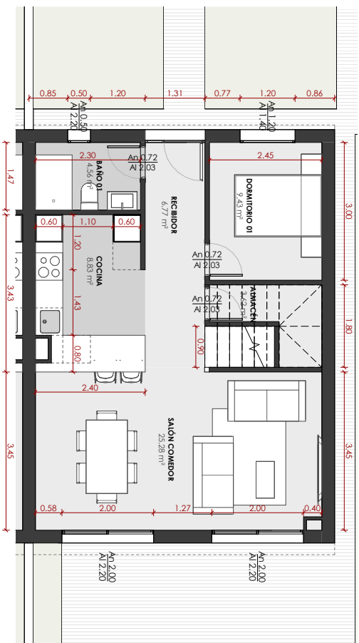
PLANTA BAJA E-1175
