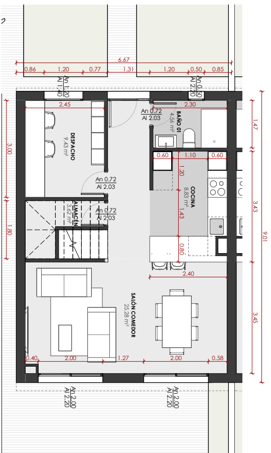
PLANTA BAJA E-1/75
